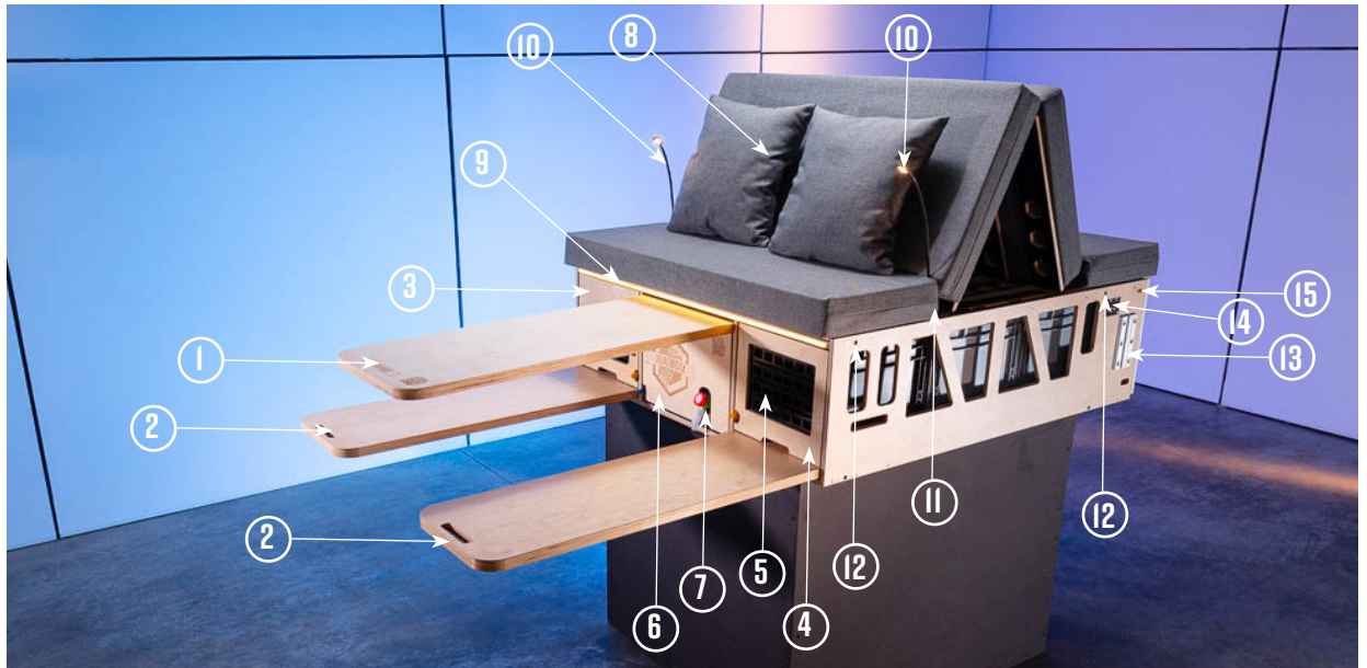
Übersicht: Fahrzeugaußenseite
